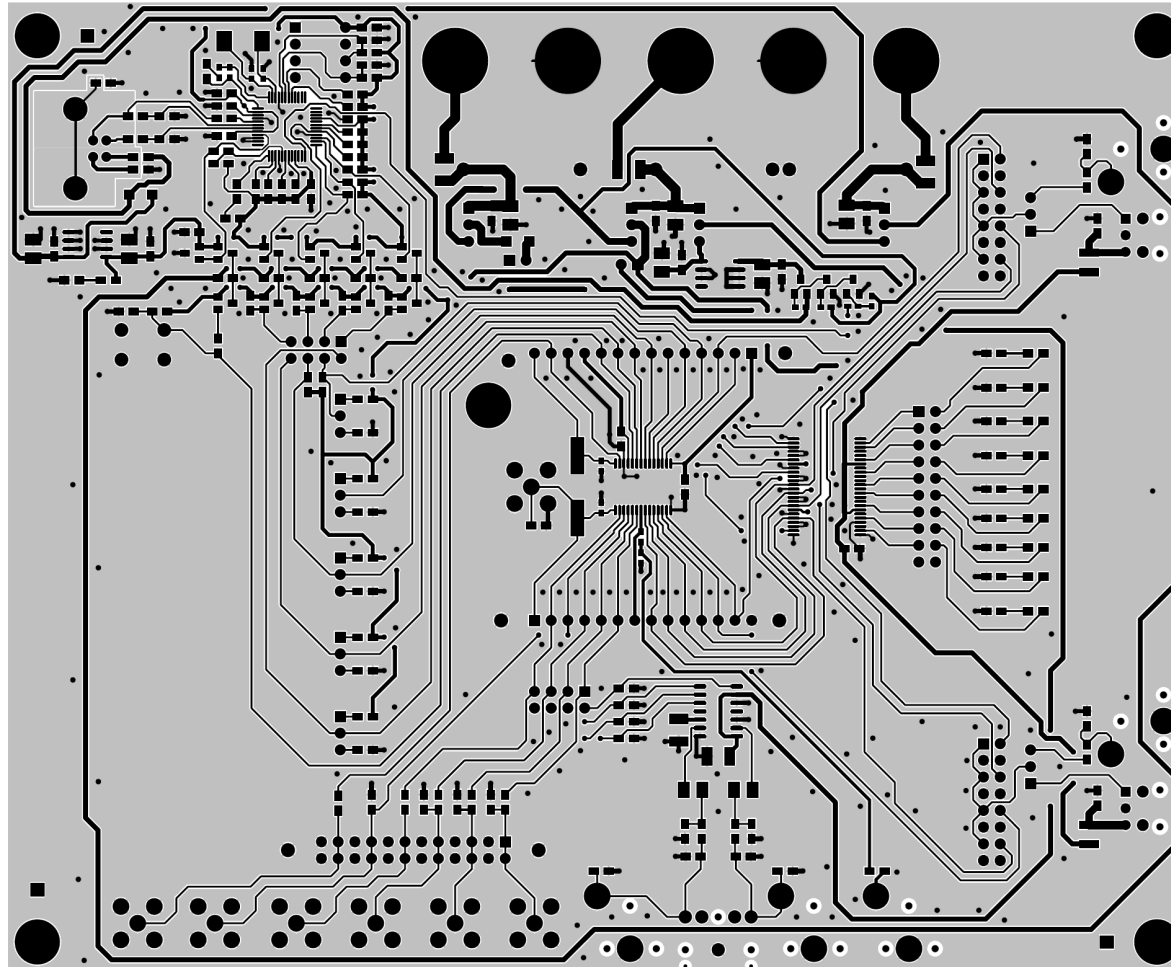
LAYER 1 TOP COPPER
