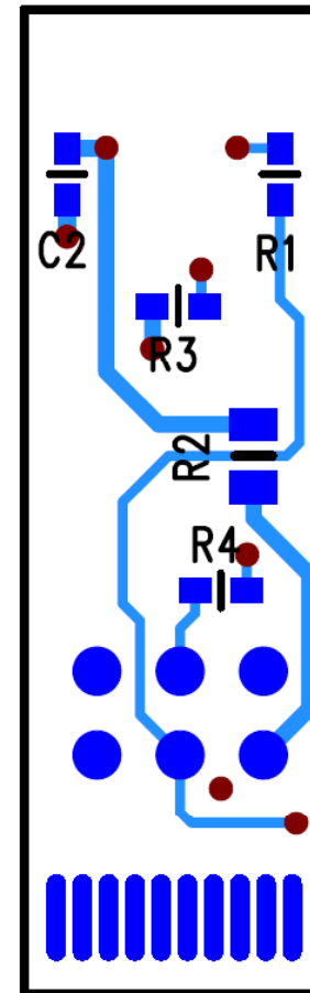
Layer 3: Copper
